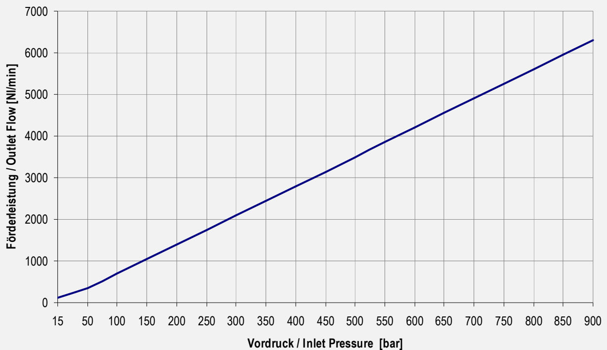
Leistungsdiagramm HDLE 30 mit doppeltem Hub Performance Graph HDLE 30 with double displacement volume
